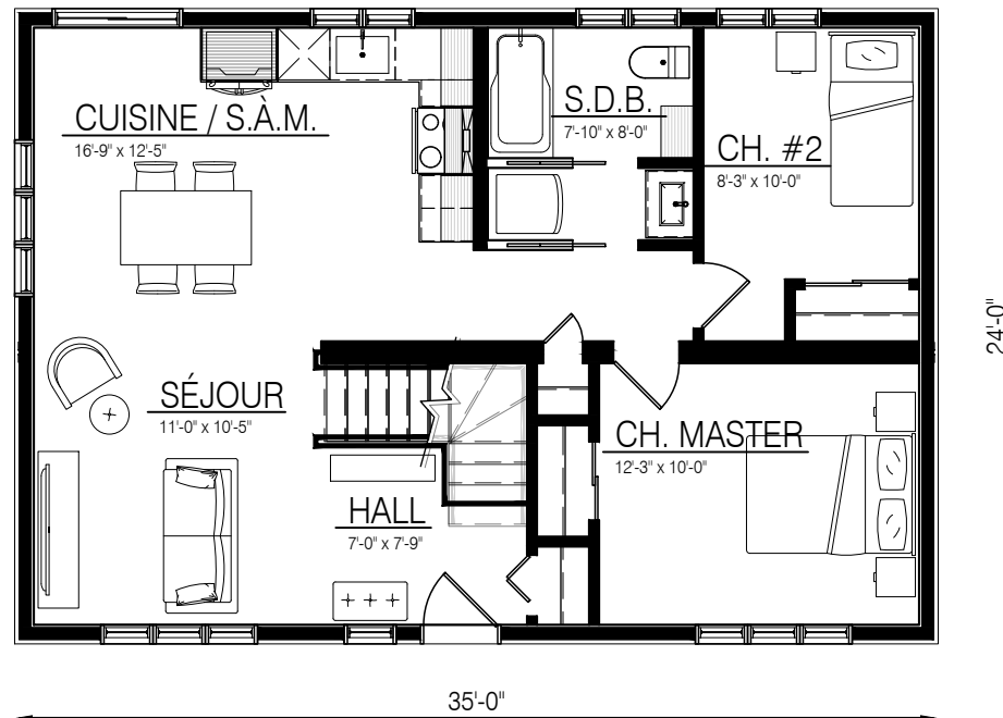
REZ-DE-CHAUSSÉE
